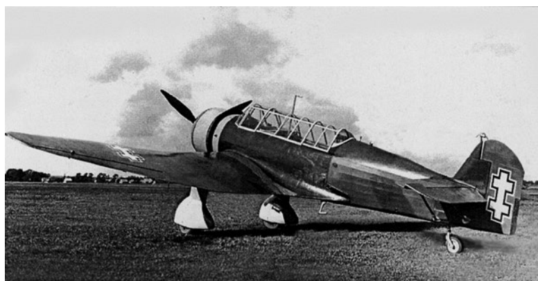
Легкий бомбардировщик ANBO-VIII конструкции генерала Антанаса Густайтиса, изготовленный в каунасских военно-авиационных мастерских (1939)
