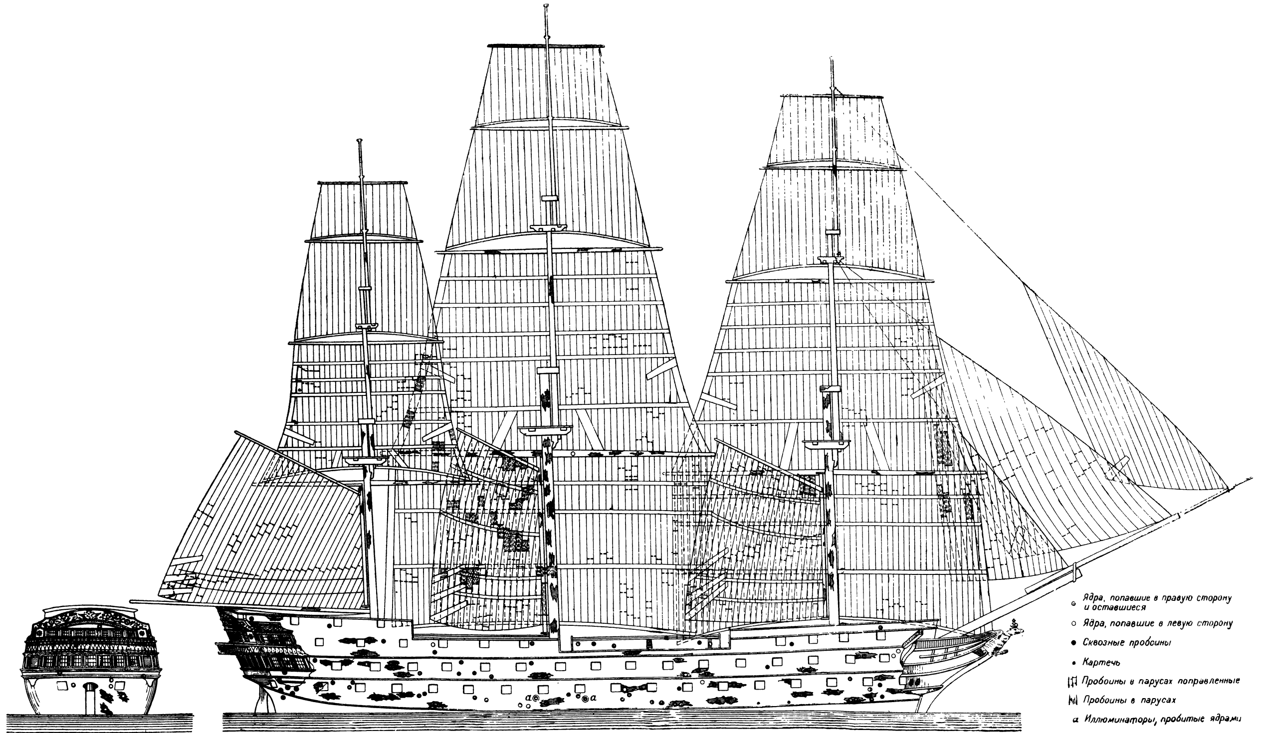
Чертеж линейного корабля «Императрица Мария», на котором держал флаг П. С. Нахимов, с указанием повреждений, полученных кораблем в Синопском сражении
