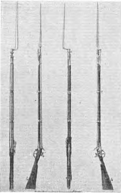
Драгунское ружье, утвержденное 30 Юня 1834 г.
