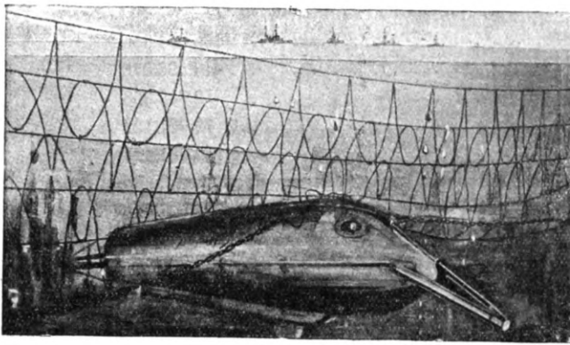
Немецкая субмарина, проходящая через заградительную сеть.
