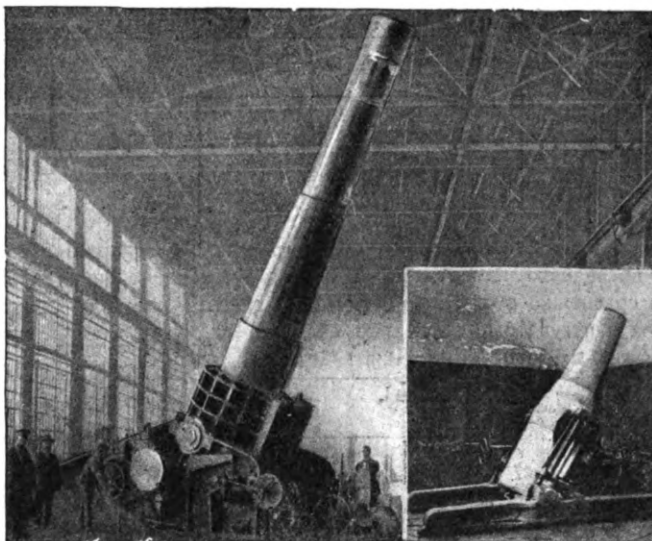
Американская 16 дм. гаубица, изготовленная во время войны, и довоенная 12 дм. осадная гаубица (в прав. углу).
