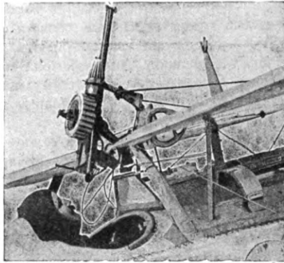
Установка пулемета на самолете.
