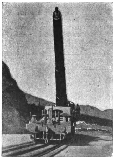
14 дм. дальнобойная пушка на ж.-д. установке.
