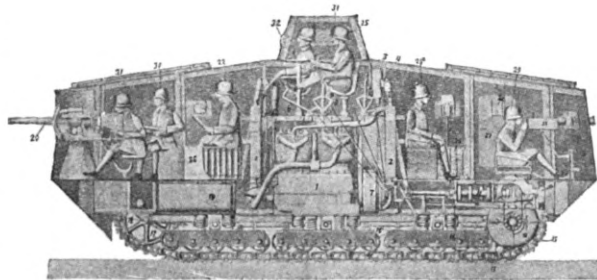
Немецкий тяжелый танк в разрезе.
