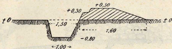
Японскій окопъ для стрѣльбы стоя.
