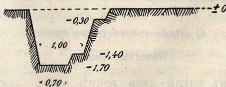
Русскіе окопы для стрѣльбы стоя.
