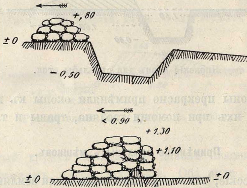
Японскіе окопы изъ земляныхъ мѣшковъ.
