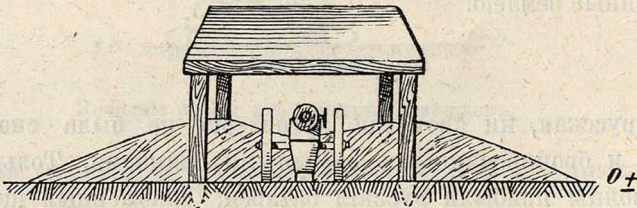
Видъ закрытаго орудійнаго окопа свади.
