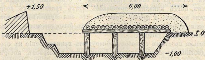
Русскій блиндажъ, устроенный въ опорномъ пунктѣ.
