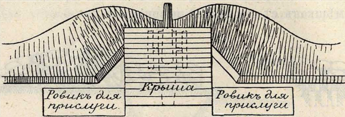
Русскій орудійный окопъ съ крышею.
