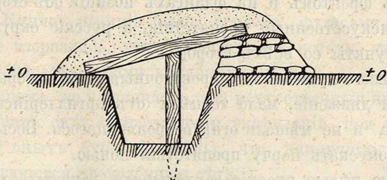
Русскій блиндажъ съ бойницами.
