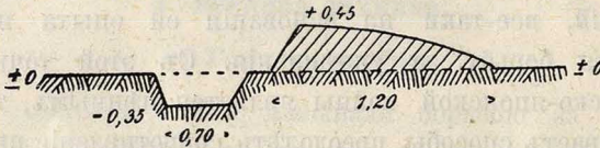
Русскій окопъ для стрѣльбы съ колѣна.
